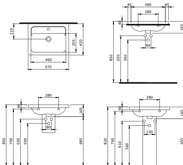
1004-001-0126 Taormina Pro Waschtisch 57 cm Taormina Pro Lavabo 57 cm Taormina Pro Wastafel 57 cm
